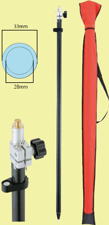
RTK ポール
