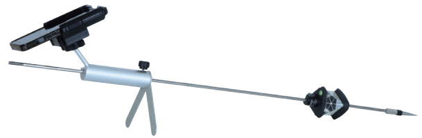
プレート型三脚がスマートフォンとプリズムを保護
