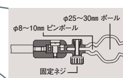
必要な長さまでアームがスライド可能 (MPPS II)
