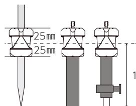
ピンボール プリズムボール スピゴットタイプ
