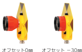
オフセット0mm オフセット -30mm
