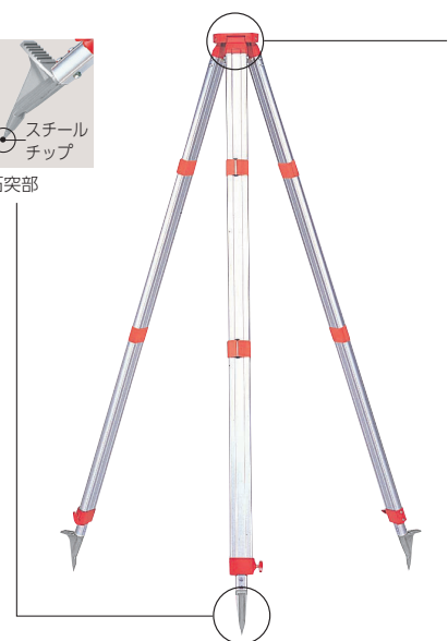
平面脚頭定芯棒 5/8インチ
