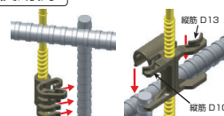
①ワンタッチ取り付け
