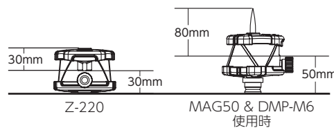
MAG50 上部：φ6mm凸 下部：5/8インチ メネジ
