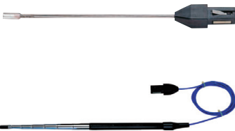
伸縮ロッド付空気センサ TA410-3DX -50~200℃ コード長 / 140cm 収納~最長 / 23cm~110cm
