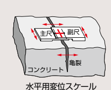
水平用変位スケール
