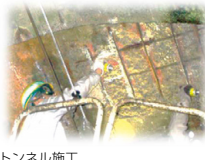
トンネル施工
